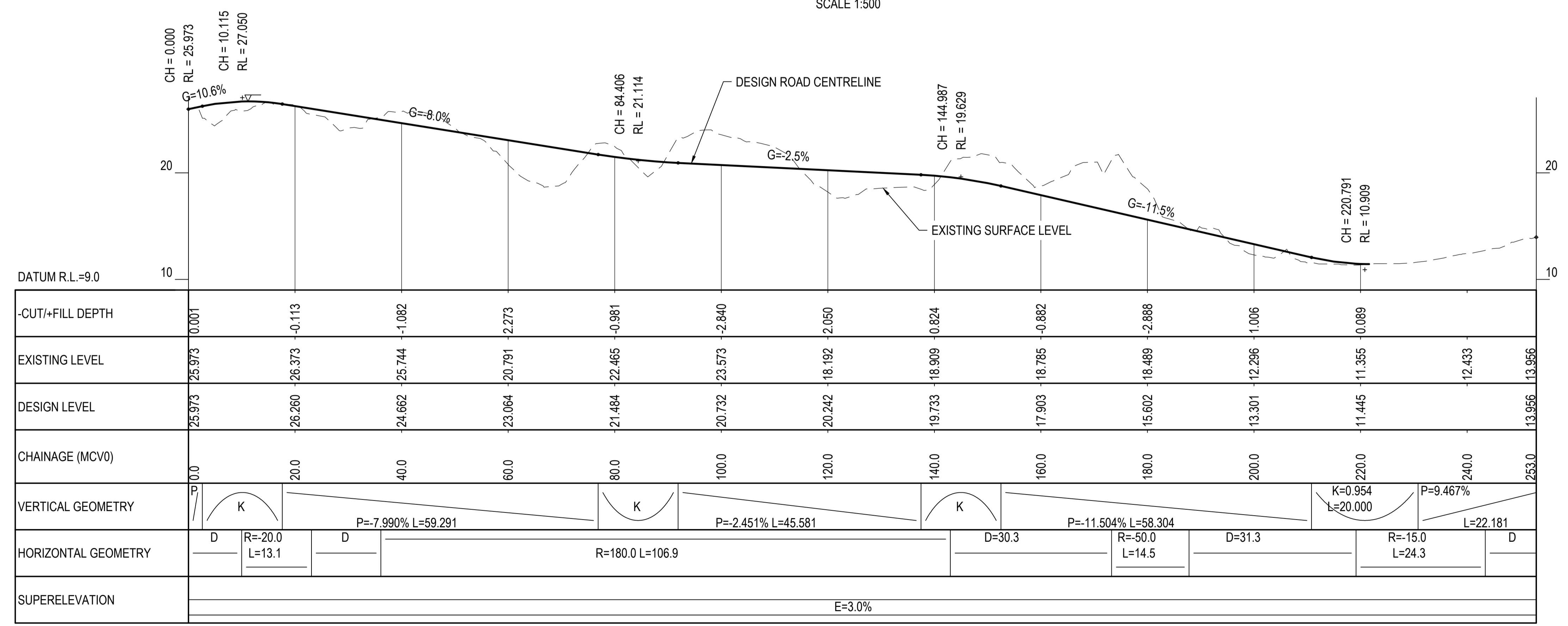
LONGITUDINAL SECTION - ROAD MCV0 HORZ 1:500 VERT 1:250
